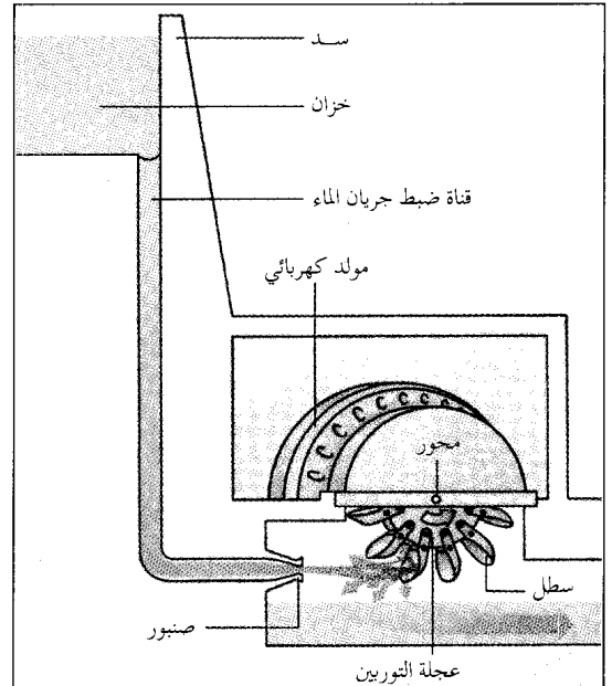
التوربين المائي يديره الماء الساقط من مكان مرتفع عبر أنبوب أو أي قناة أخرى. توربين بلتون المبين في الشكل يدير مولدًا كهربائيًا في مصنع للورق.
