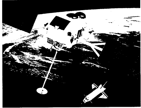
مرصد كومبتون لأشعة جاما. قمر صناعي أطلق في سنة ١٩٩١م وهو يحمل بعض الأجهزة اسمها الملائكات للكشف عن أشعة جاما وقياس كثافتها وتحديد مصادرهما.
