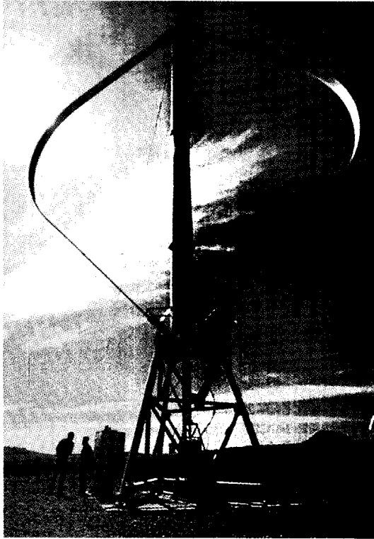
توربين داريو الهوائي توربين هوائي ذو محور عمودي. فعالية توربين داريو الهوائي عالية جداً فباستطاعته أن يستفيد من حركة الريح في أي اتجاه.
