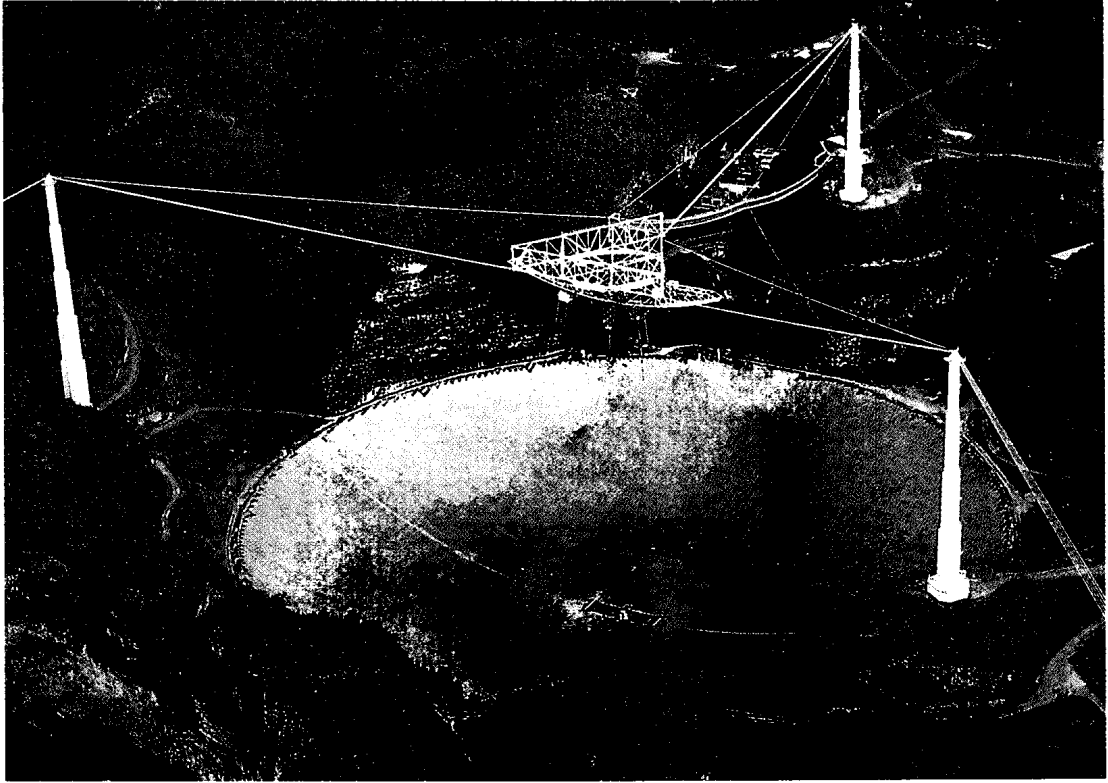
تلسكوب لاسلكي ضخم أنشئ في الهضاب قرب أرسيبو، بورتوريكو. يبلغ قطر عاكس التلسكوب ٣٠٥م، وتغطيه من الداخل صفائح الألومنيوم. تعكس هذه الصفائح الموجات اللاسلكية (الراديوية) الآتية من الفضاء في الهوائي المعلق فوق العاكس.
