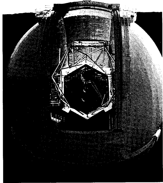
التلسكوب الكيكي الموجود في ماونا كاي في جزيرة هاواي له مرآة كبيرة بإقطاعات قطرها ١٠ أمتار. وتتكون المرآة من ٣٦ قطعة.
