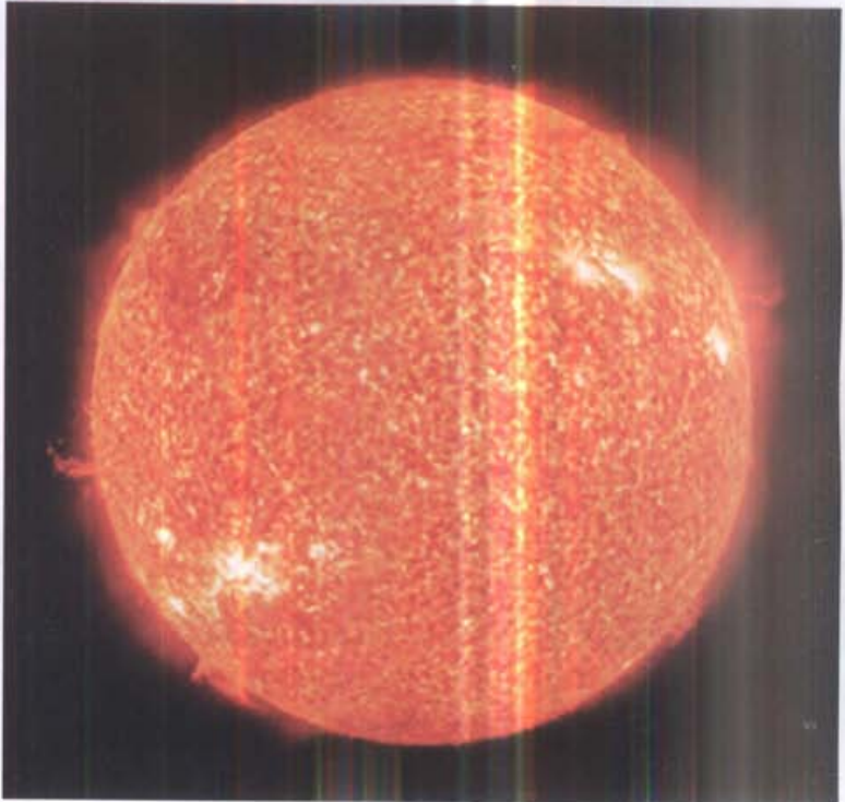
Sun
